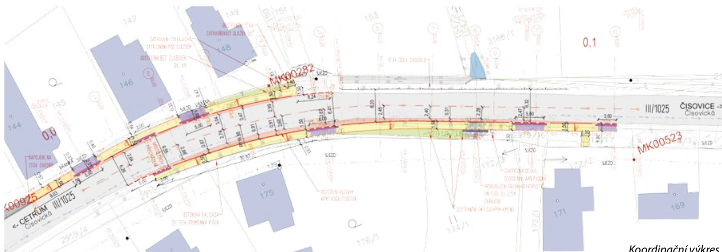
Koordinální výkres
