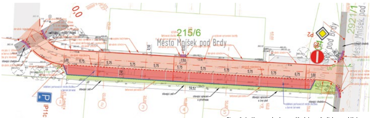
Situační výkres – plocha za dětským střediskem a lékárnou
